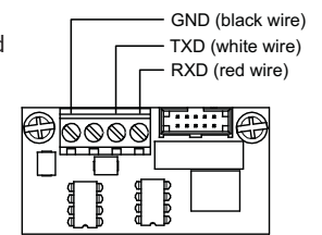
SA-232 wiring
